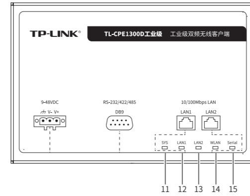
TL-CPE1300D工业级 顶面板示意图
